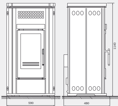
► Stove 51 P
