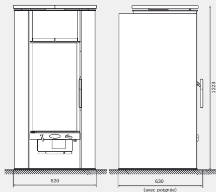
► Stove 41 W
