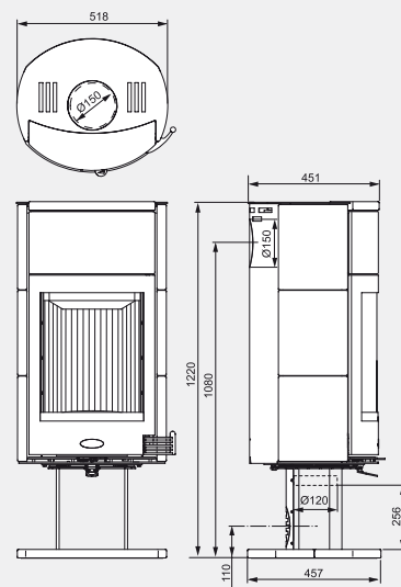
► Stove 33
