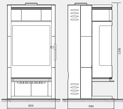
► Stove 31
