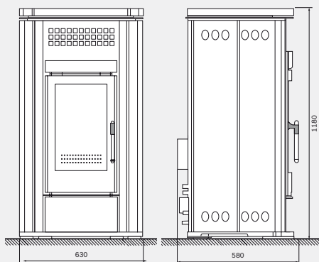
► Stove 52 PW
