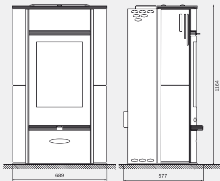
► Stove 32
